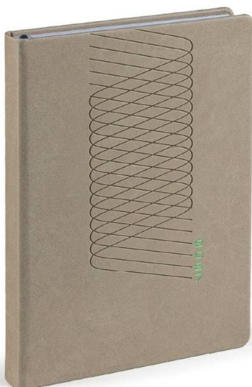
ZK 12 · Interferencja
