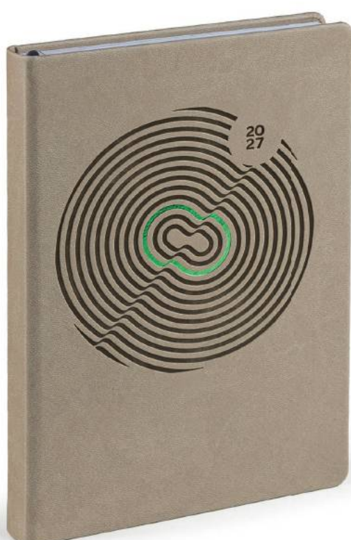
ZK 04 · Echo
