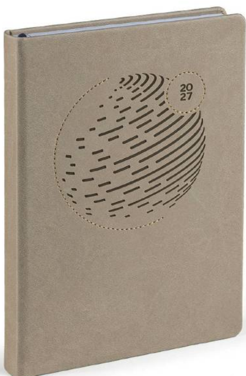
ZK 03 · Planeta
