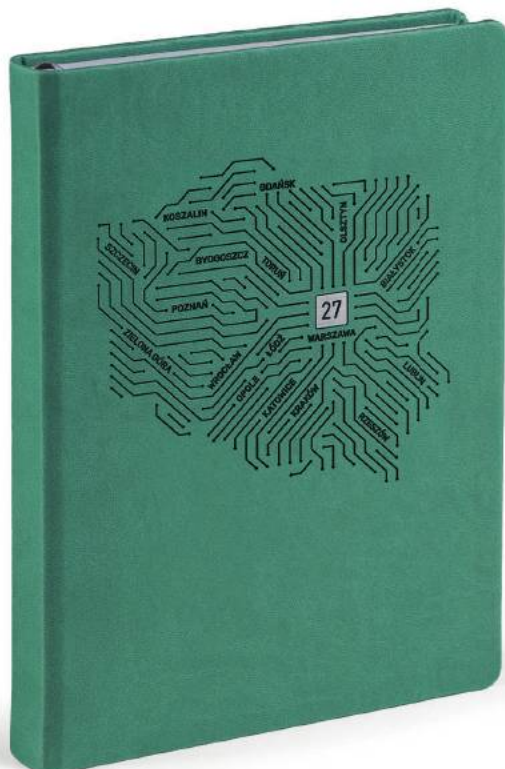
ZK 08 · Polska
